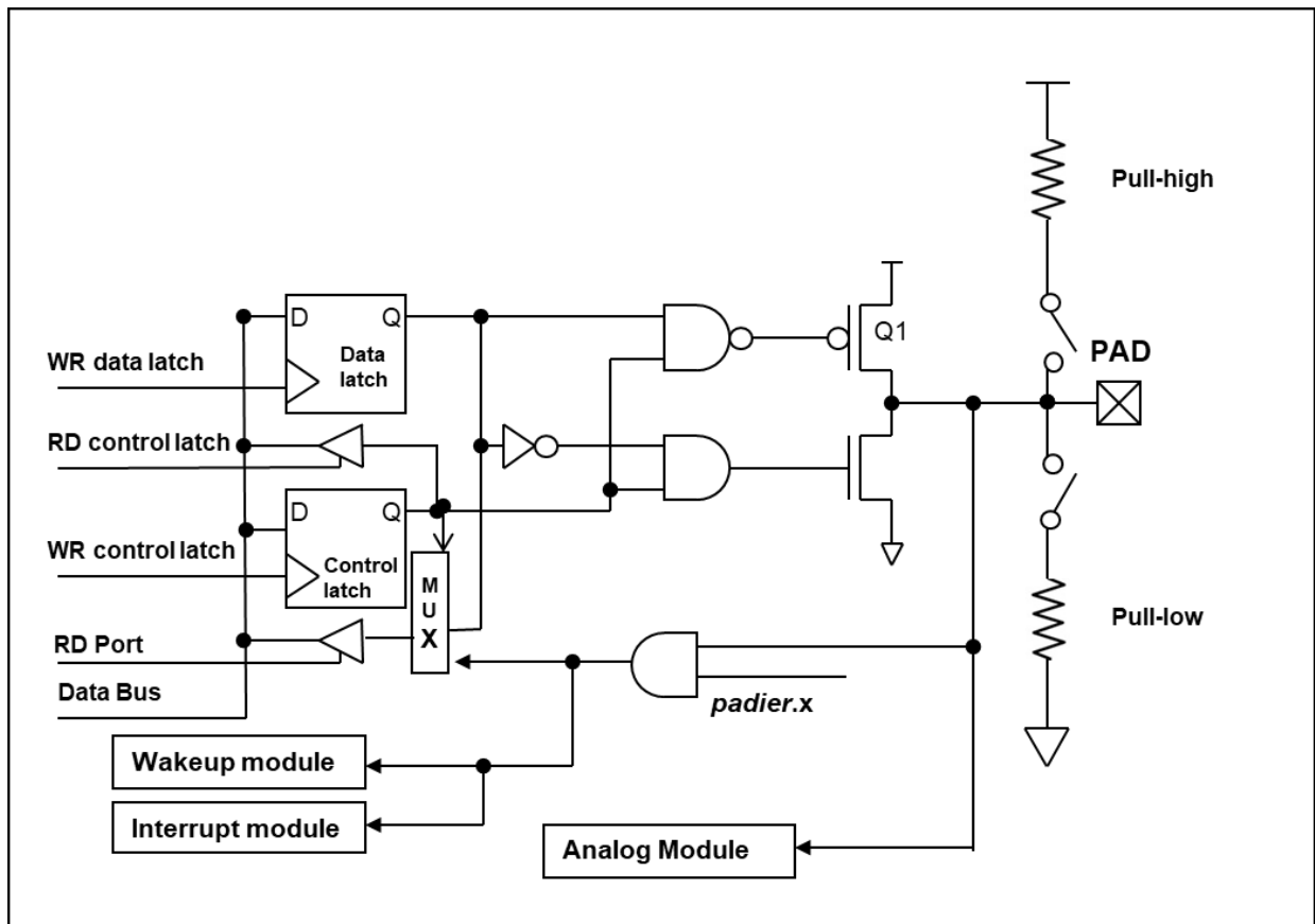
图 17: IO 引脚缓冲区硬件图
